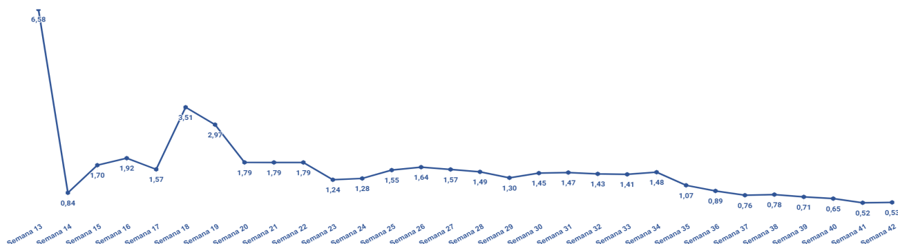
Gráfico 5. R_0 * por semana epidemiológica em Palmas-TO, 2020.
