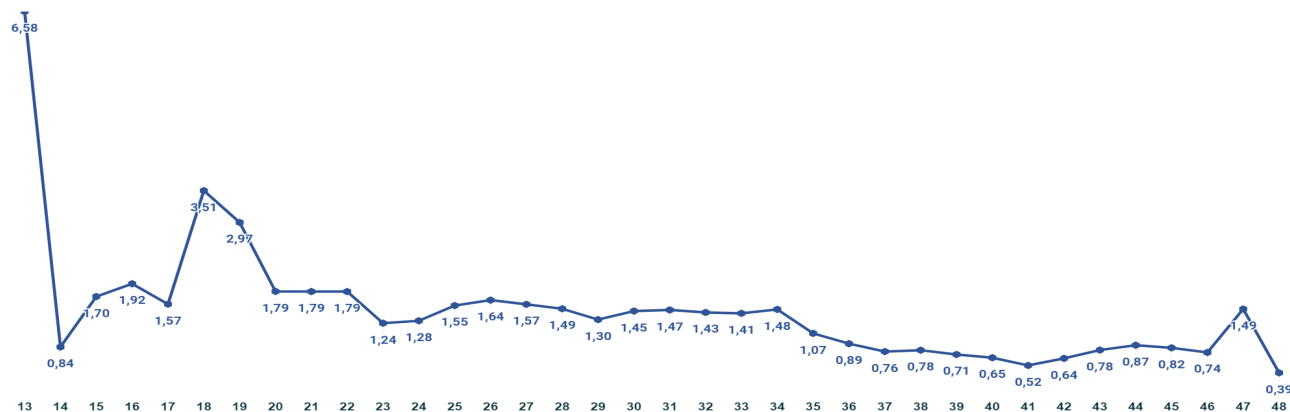
Gráfico 5. Média do R_0^* por semana epidemiológica em Palmas-TO, 2020.
