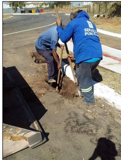
Desentupimento de Boca de Lobo e reparo de grelha em rotatória. Comumente as grelhas de concreto localizadas em rotatórias da cidade são avariadas pelo tráfego dos automóveis
