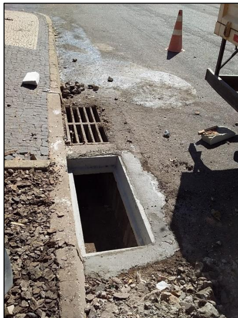
Desobstrução da caixa receptora da boca de lobo e substituição da grelha
