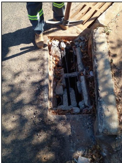
Reparo da caixa da boca de lobo e da respectiva grelha
